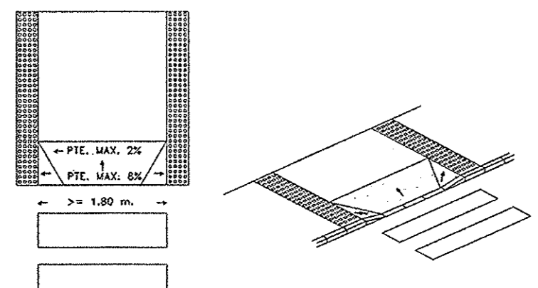
DETALLE DE PASO DE PEATONES
